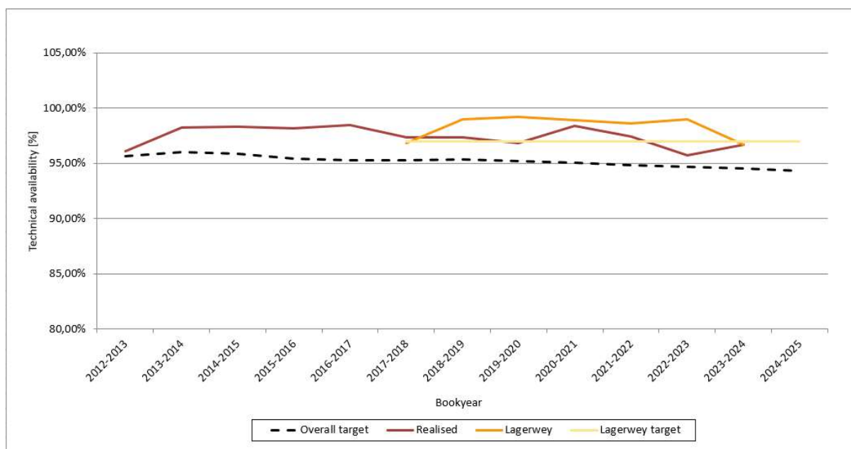
Figuur 16: Technische beschikbaarheid van de Lagerwey-turbines (Goeiende) sinds 2012
