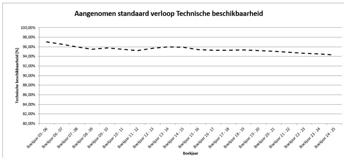
Figuur 11: Aangenomen standaard verloop technische beschikbaarheid
