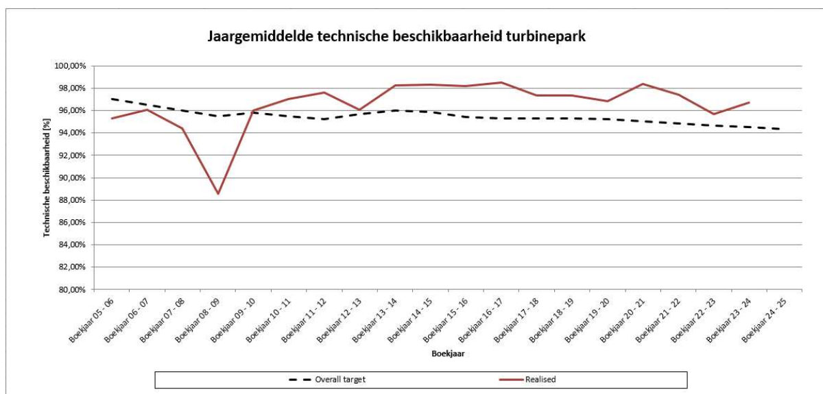
Figuur 12: Jaargemiddelde en doelstelling technische beschikbaarheid turbinepark
